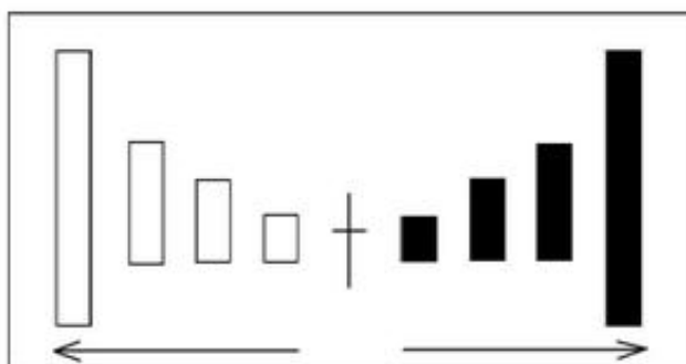
K线长度变化与动力转化图
